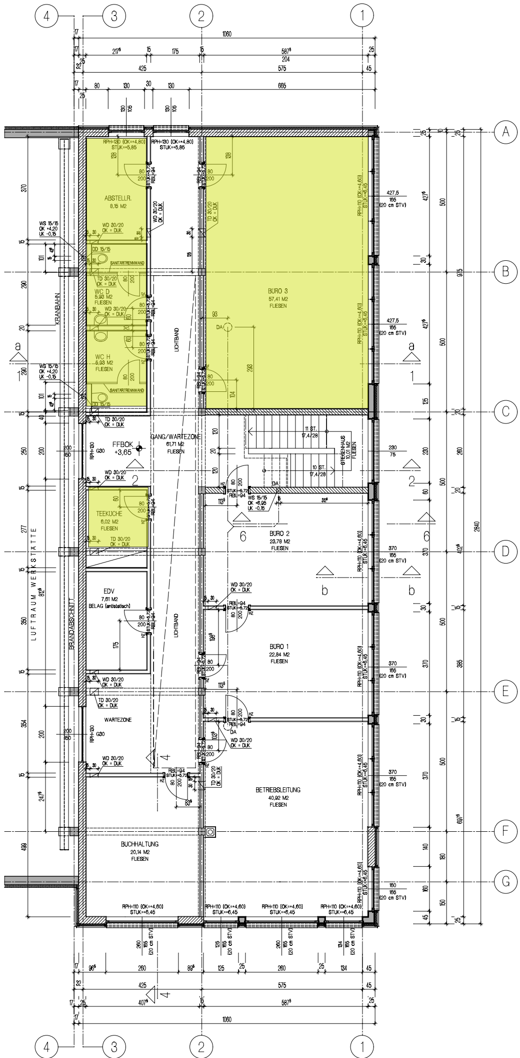
GRUNDRISS OBERGESCHOSS
